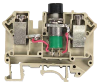
Bornes Customizados com botão de teste
