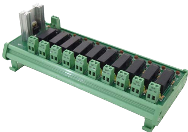
Interface para Proteção de Câmeras
